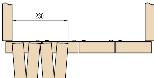
SISTEMA A QUATTRO ANTE / SYSTEM FOR FOUR DOORS
